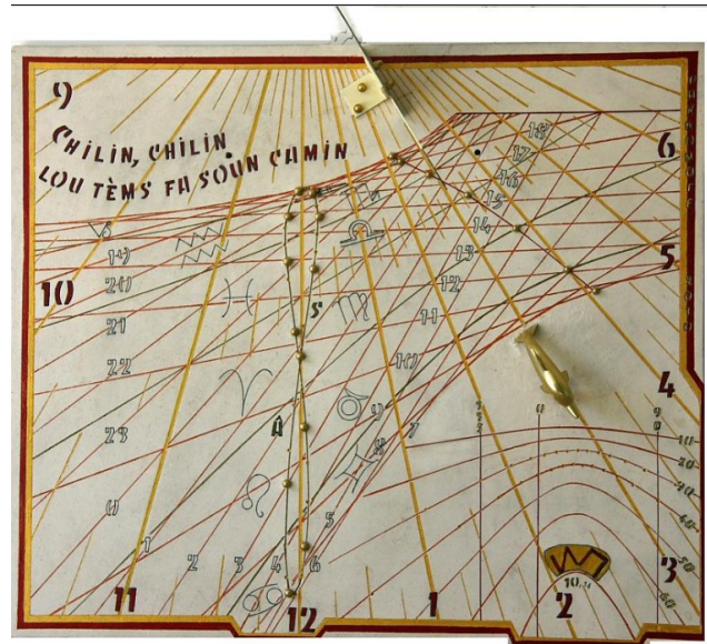
Cadran bifilaire et cadran à heures sidérales
