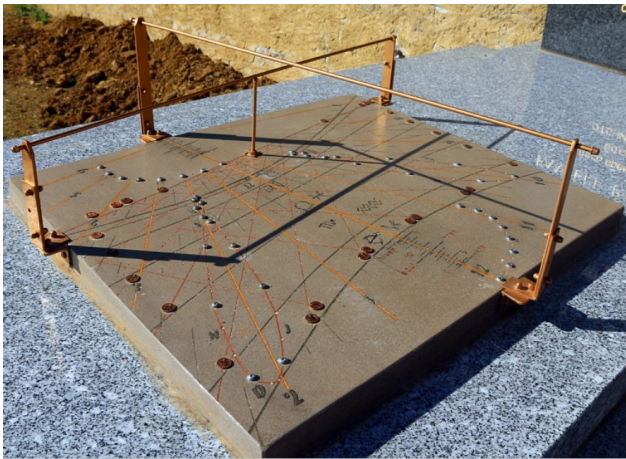
Cadran bifilaire et cadran à heures sidérales
